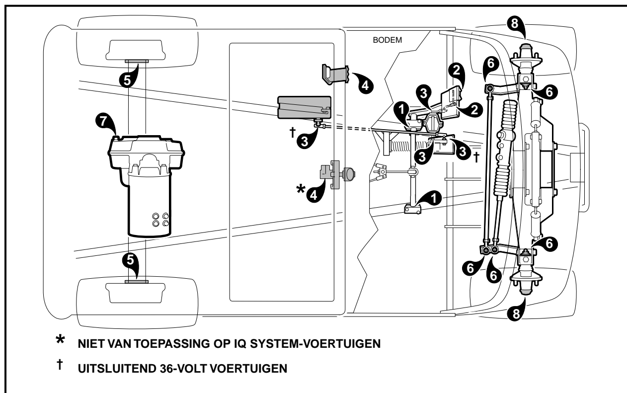
Figuur 11 Smeerpunten
