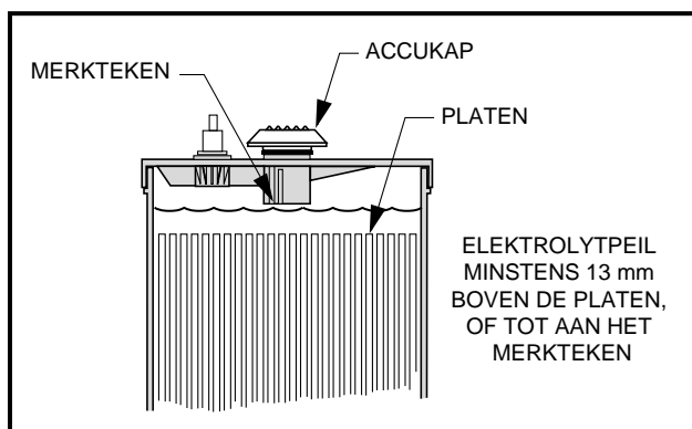
Figuur 12 Elektrolytpeil van accu
