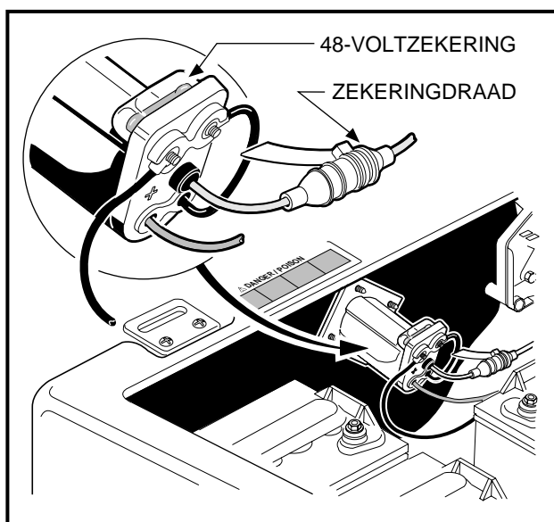
Figuur 16 Zekering stopcontact voor 48-volt voertuig
